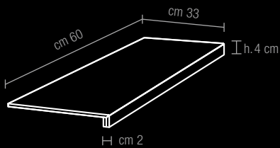
Gradone (assemblato)
